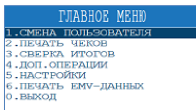
Рис.6 – Меню кассира
